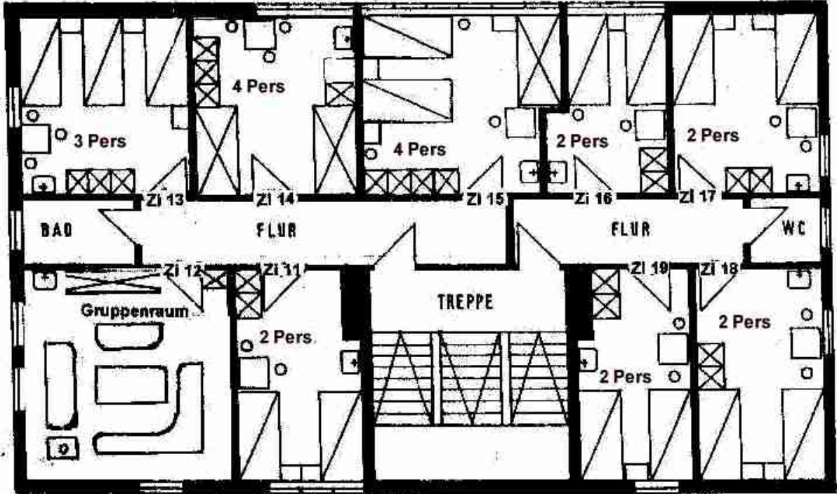
2. Obergeschoss
